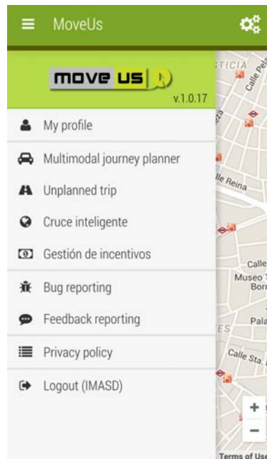
Figura 18 - Aplicación MoveUs
